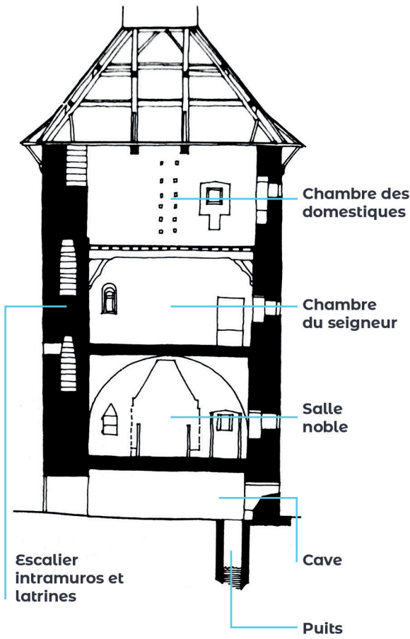
Coupe verticale de la tour romane par L-F Génicot pour la Commission Royale des Monuments et Sites (CRMS)
